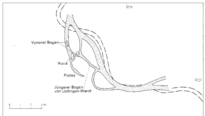
Abb. 6 Der spätrömische Rhein
