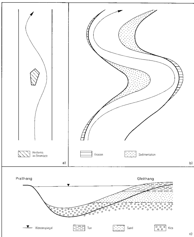
Abb. 3 Entstehung eines mäandrierenden Stroms mit seinen Ablagerungen
