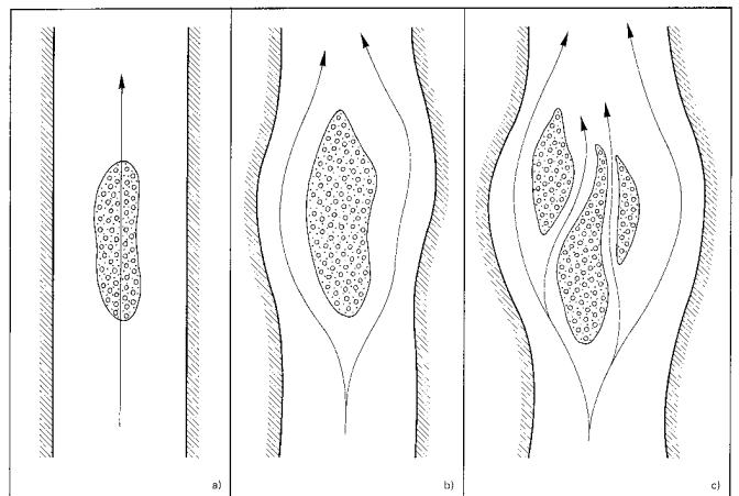
Abb. 2 Entstehung eines verwilderten Flußsystems
