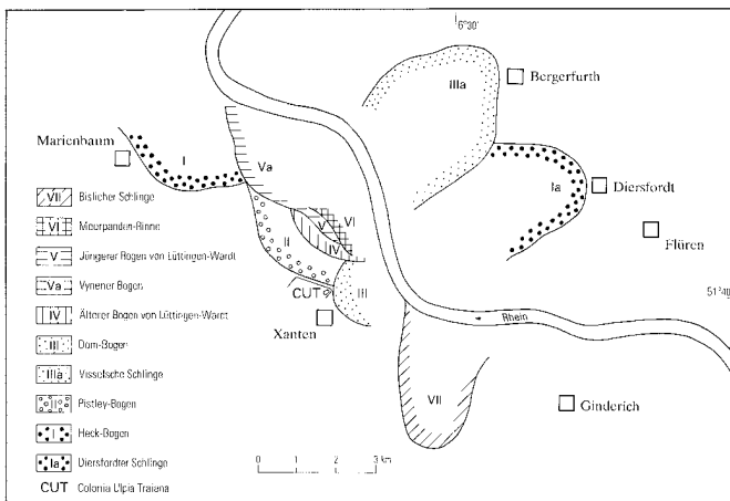
Abb. 1 Lage des Untersuchungsgebietes und Stromrinnen des Rheins
