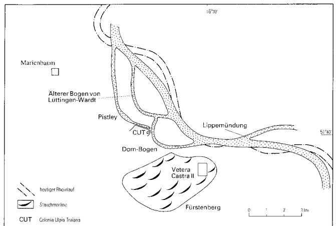
Abb. 5 Der Rhein während der frühen Römerzeit
